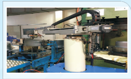
机械手作业 自動搬送 Robot Operating
